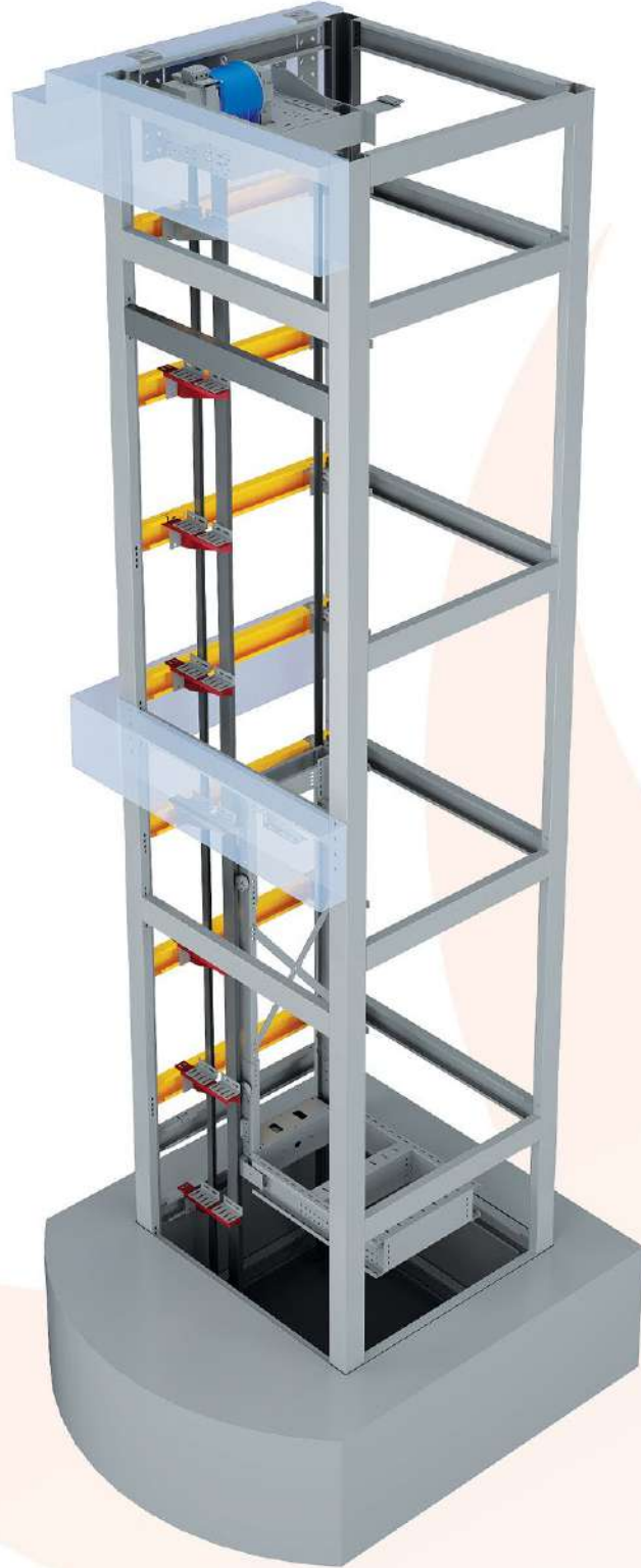
2:1 Askı MRL L Karkas Sistemi 2:1 Hanger MRL L Frame System 2:1 Вешалка (Mrl) L Каркасная Система 2:1 مصعد بدون غرفة شاصة حرف L
