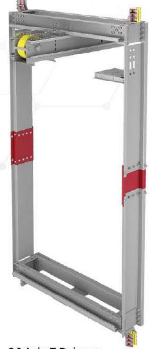
2:1 Askı T Palanga Kabin Süspansiyonu
